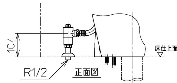
床給水仕様の場合
